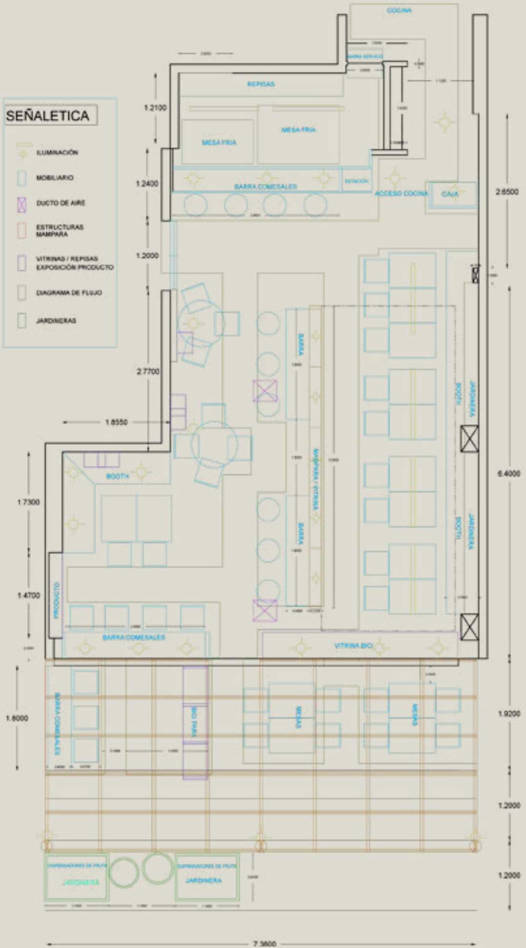
PLANO COTAS
