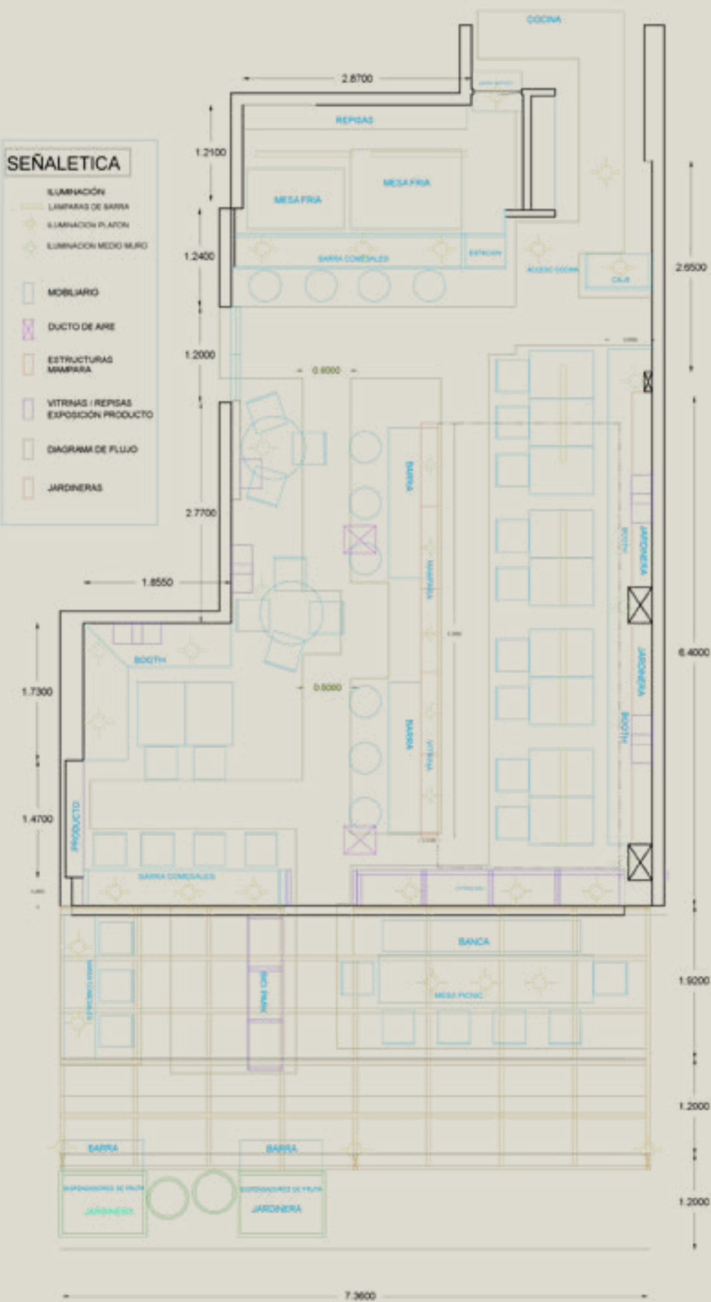
PLANO ILLUMINACION
